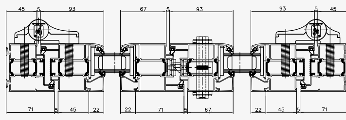
Coupe horizontale
