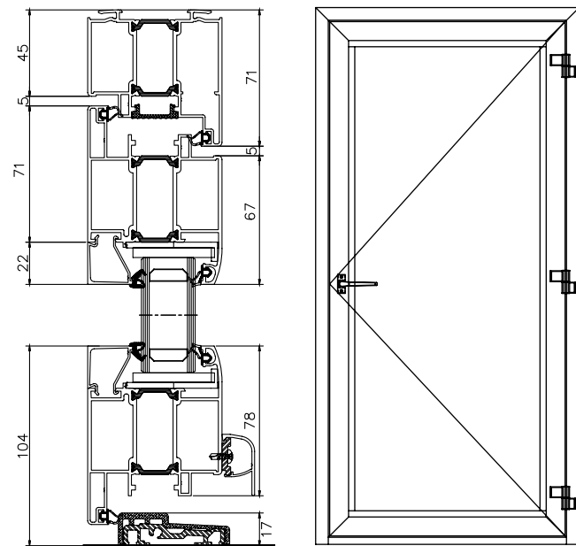
Coupe verticale
