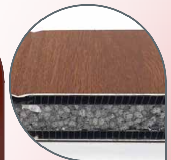
Panneau 28 mm chêne doré
