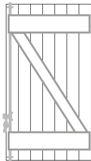
Barres avec espagnolette traversante
