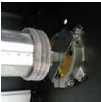
Le parachute intégré à l'axe d'enroulement coupe le moteur et bloque la porte dans sa position en cas de défaillances techniques.
