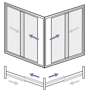
2 x 2 vantaux
