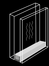
Vitrage acoustique 44.1 acoustique / 16 argon / 8 ITR
