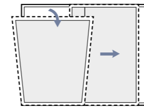
Fenêtre oscillo-couissante
