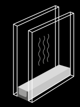
Vitrage à faible émissivité 4/16 argon / 4 ITR
