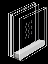
Vitrage résistance à l'effraction 44.6 / 10 argon / 4 ITR 44.6 / 12 argon / 4 ITR
